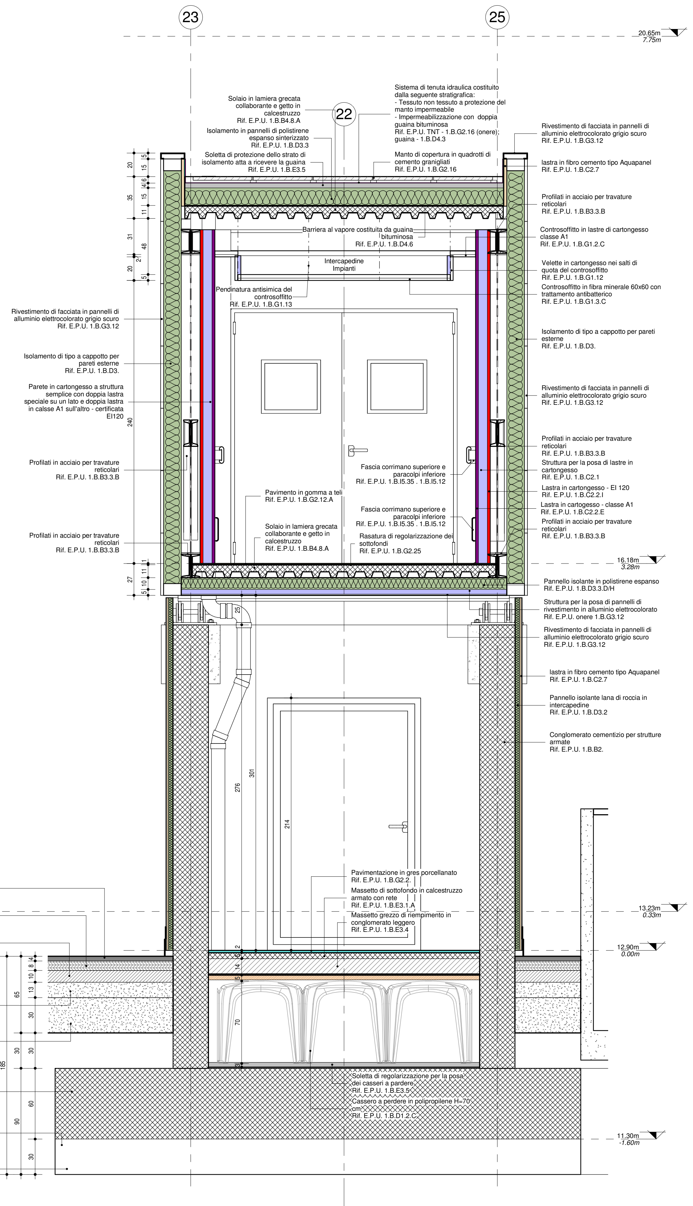
TC.1 Tunnel di collegamento - dettaglio 1 Scala: 1 : 20
