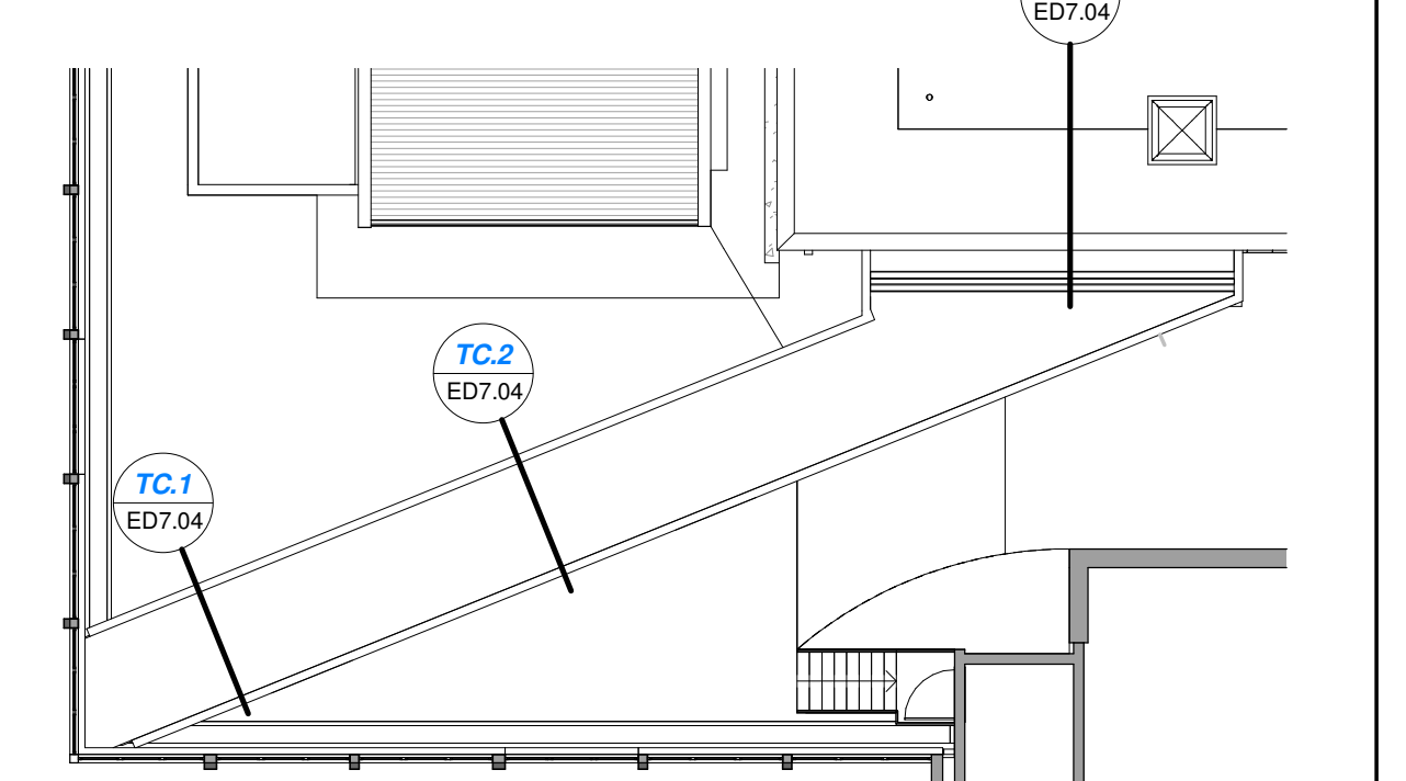
Piano Primo-Copertura 1 : 200
