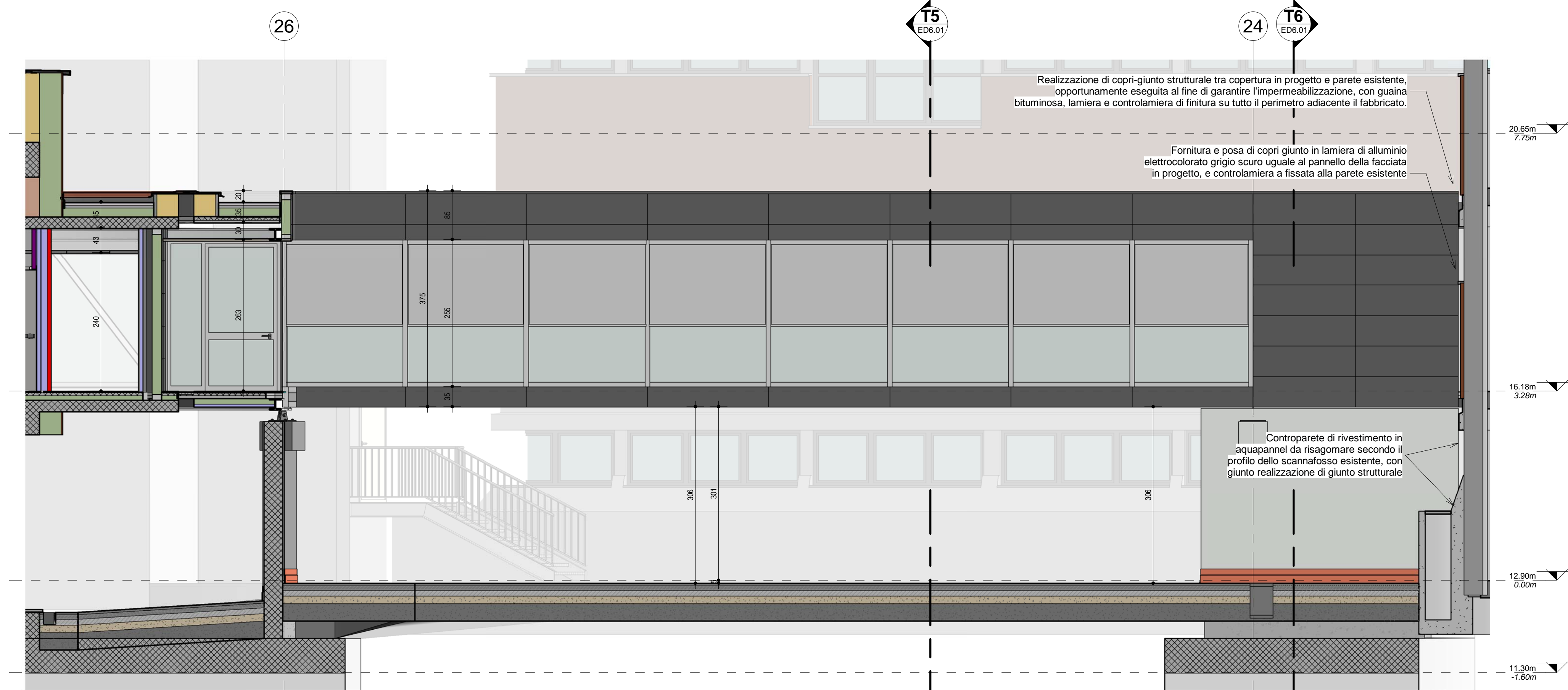
Prospetto Sud 1 : 50
