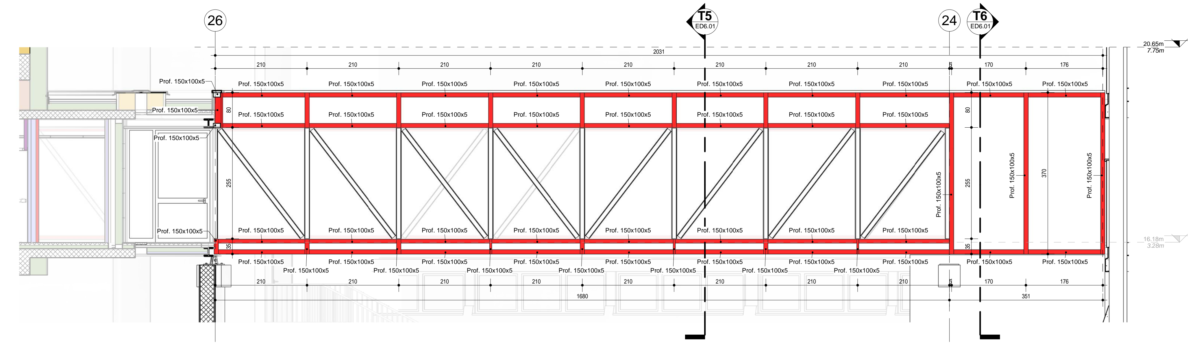
Prospetto Sud - Struttura di facciata 1 : 50
