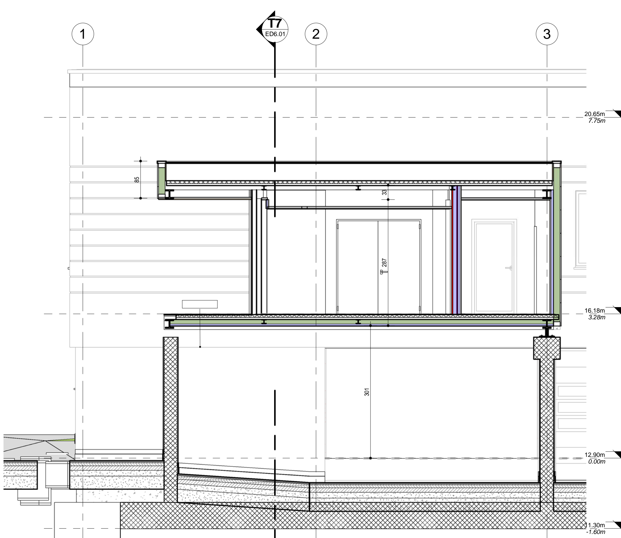
Sezione T3-T3 1 : 50
