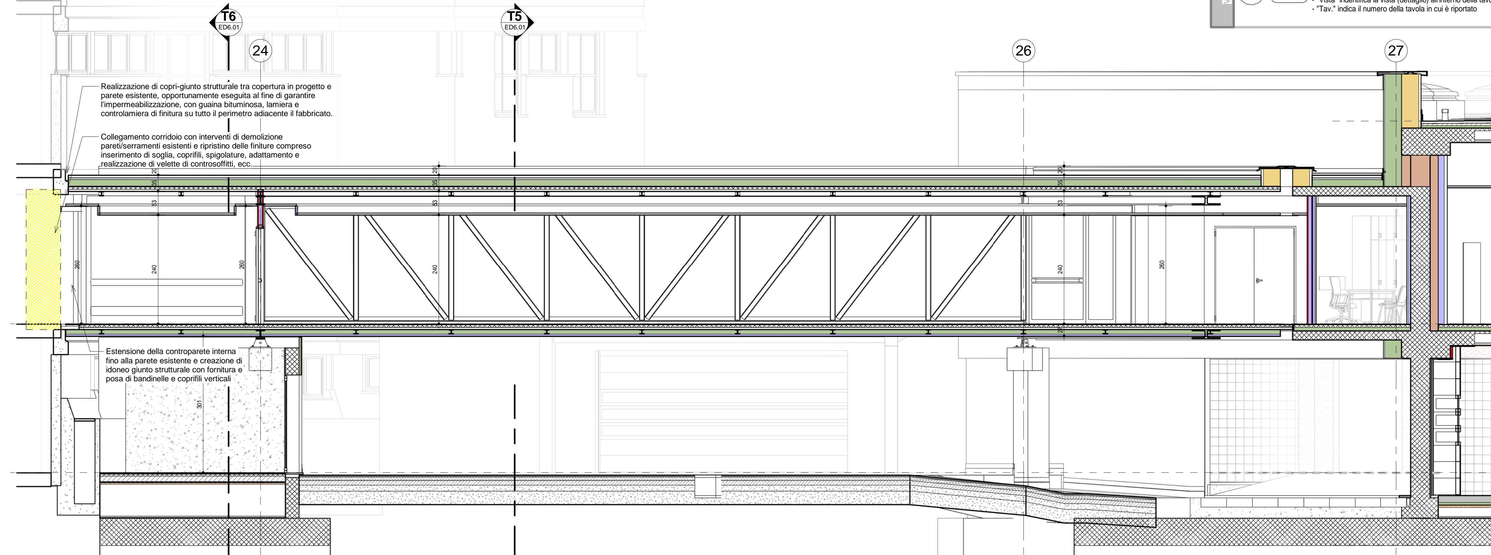
sezione T4-T4 1 : 50
