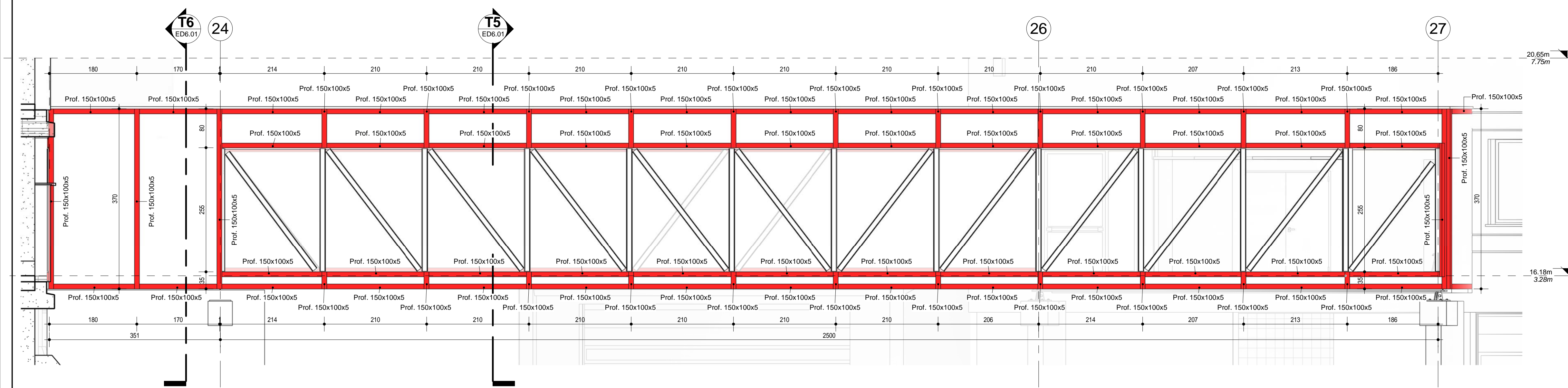
Prospetto Nord - Struttura di facciata 1 : 50
