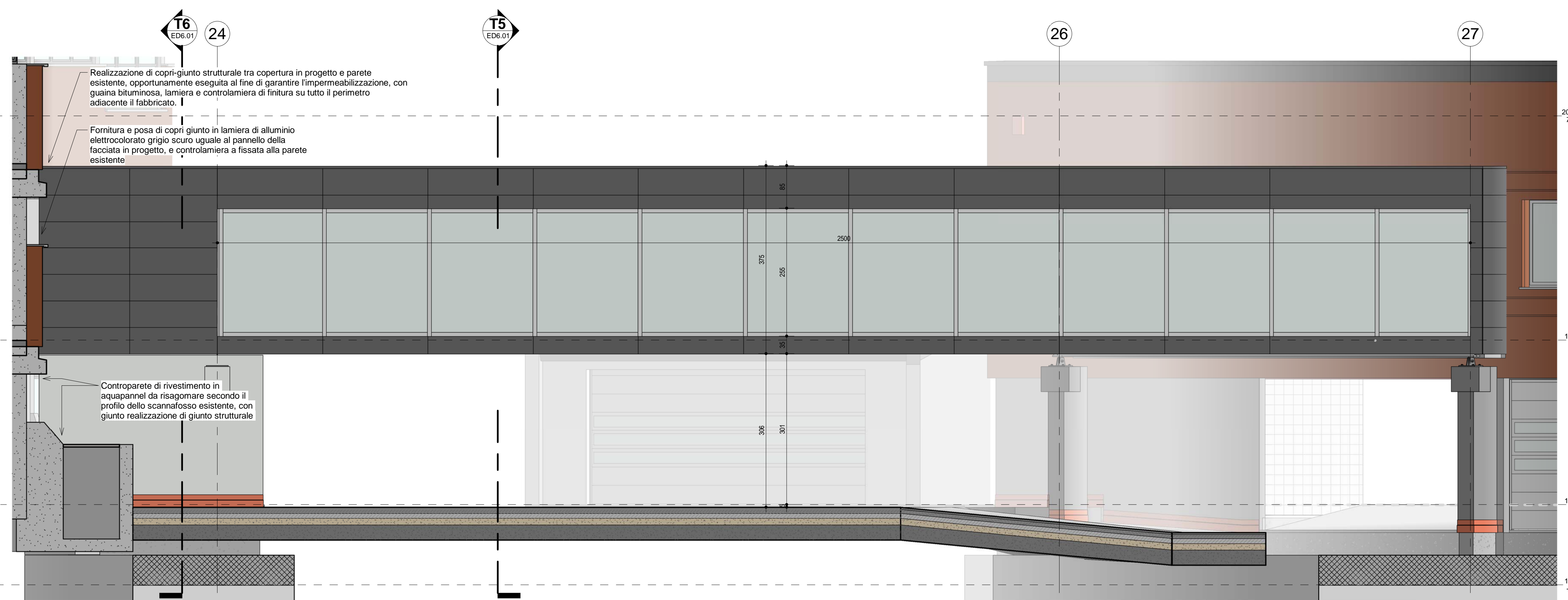
Prospetto Nord 1 : 50
