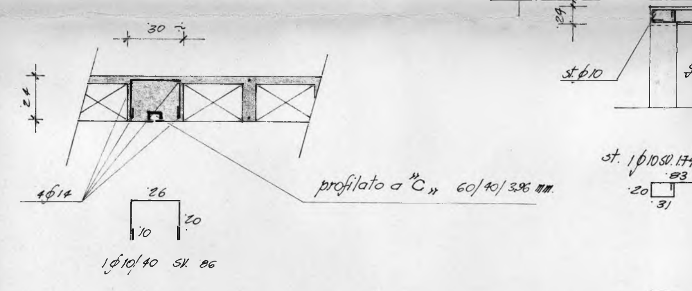
sezione tipo cordoli
