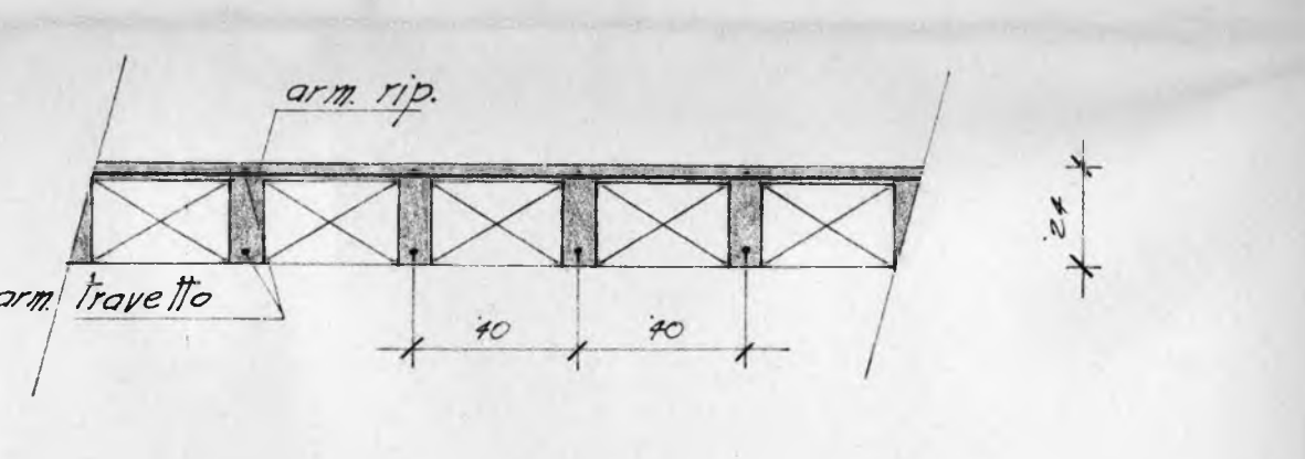
sezione tipo solaio
