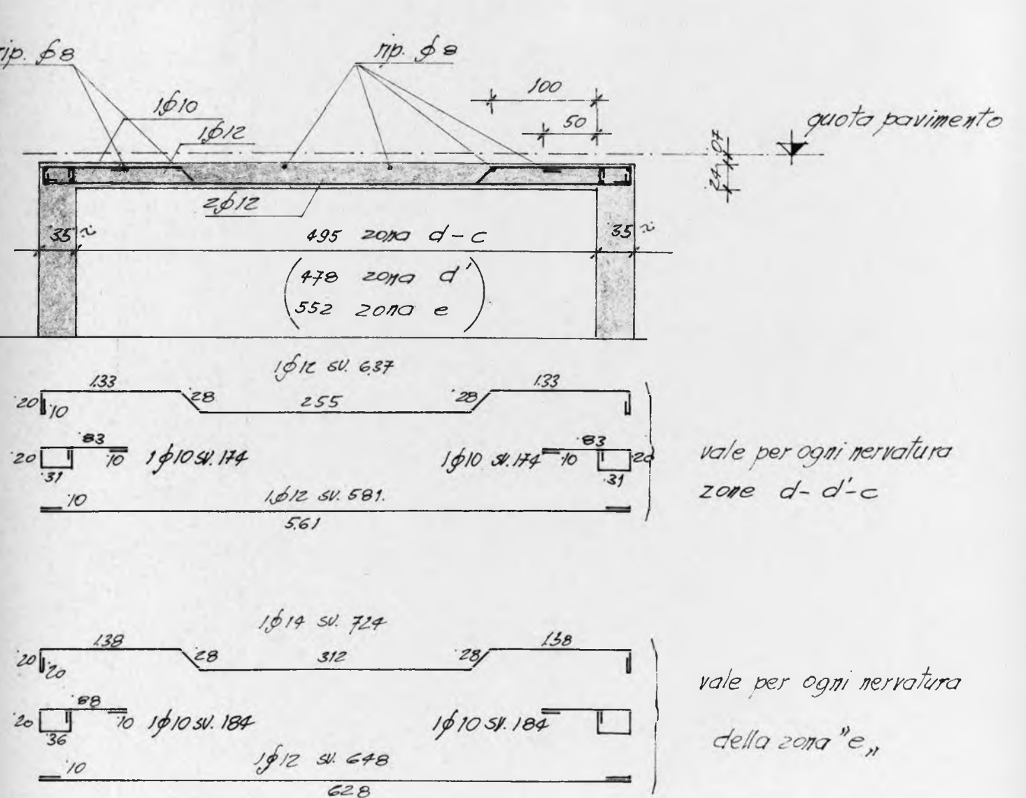
solai zona d-d'-c ad e.
