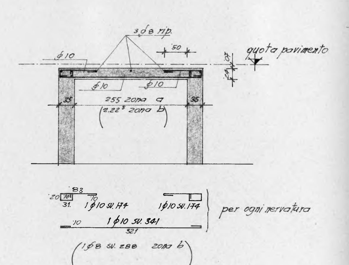
solai zona a-b
